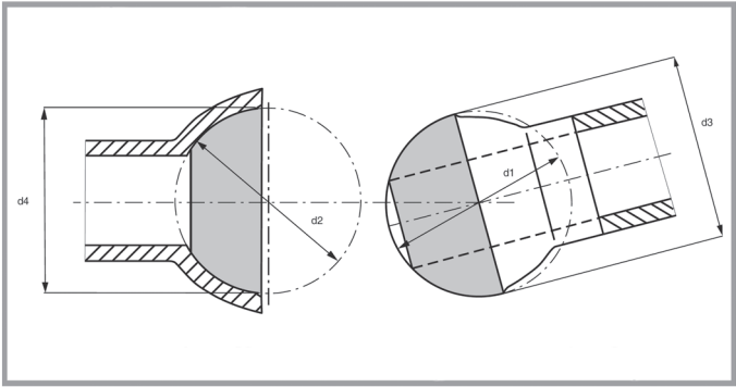
Шлиф сферический (DIN12244, 12246)
